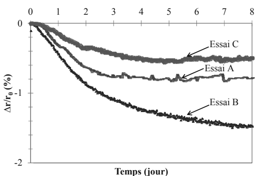
Figure 6 : Évolution des déformations latérales en fonction du mode de séchage.
