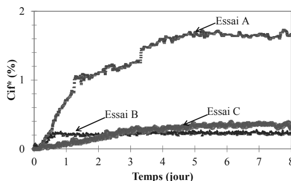
Figure 8 : Évolution du Cif^* en fonction des sollicitations hydriques.
