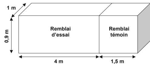
Figure 3. Dimensions du remblai R1
