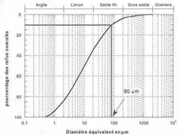
Figure 1. Courbe granulométrique de l'argile de Bavent (Alshihabi, 2002)
