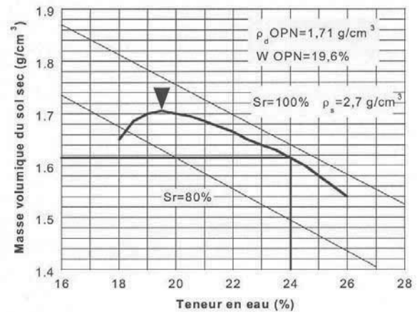
Figure 2. Courbe Proctor normal de l'argile de Bavent
