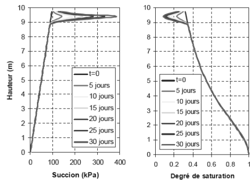
Figure 3 Variations du profil de la succion et du degré de saturation
