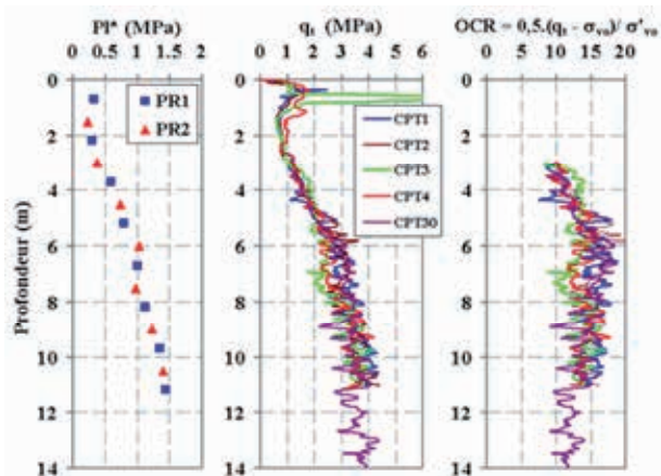
Figure 2. Profils de pression limite nette pressiométrique pl*, de résistance au cône q t et de l'OCR sur le site de Merville
