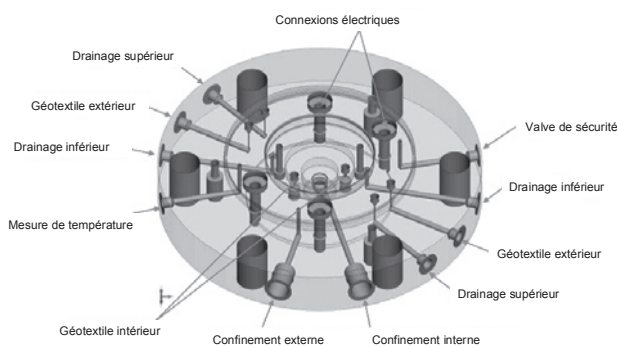
Figure 2. Schéma de l'embase de la cellule.
