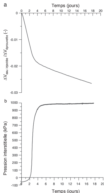
Figure 4. Resaturation de l'éprouvette d'argile de Boom
