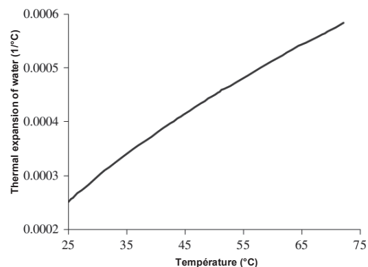
Figure 7. Variations du coefficient de pressurisation thermique de l'eau sous 4 MPa (Spang 2002)
