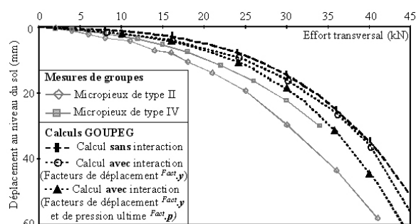
Figure 10. Essais de chargement transversal des groupes de micropieux de type II et de type IV. Courbes effort-déplacement issues des mesures et des calculs à l'aide du logiciel GOUPEG-3D.
