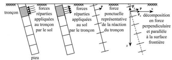
Figure 6. Passage des forces réparties calculées par le logiciel GOUPEG aux forces ponctuelles des équations de Mindlin.
