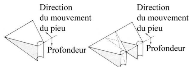
Figure 2. Zones de chevauchement des contraintes de cisaillement de la rangée « avant » (Brown et al., 1988)
