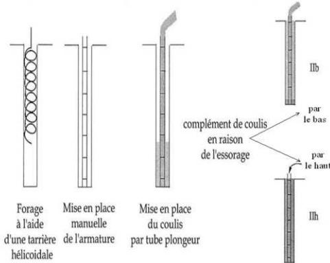
Figure 7. Réalisation des micropieux de type IIb et IIh.
