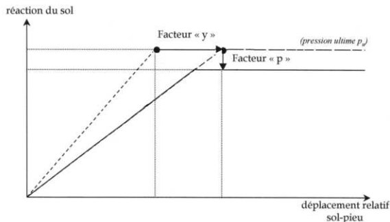
Figure 4. Modélisation de la prise en compte de l'effet de groupe par modification des courbes « P-y » par l'association de facteurs correcteurs de déplacement « \langle y \rangle » et de pression limite « \langle p \rangle ».
