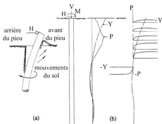
Figure 1. a) Comportement du sol autour du pieu au voisinage du terrain naturel (T.N.) (Broms, 1964) b) Réponse « P-y » d'un pieu sous un chargement transversal hypothétique (O'Neill et al., 1985) V : effort axial en tête ; H : effort transversal en tête de pieu ; M : moment en tête de pieu ; Y : déplacement dans la direction transversale ; P : réaction du sol dans la direction transversale.
