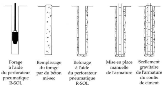
Figure 8. Réalisation des micropieux R-SOL.
