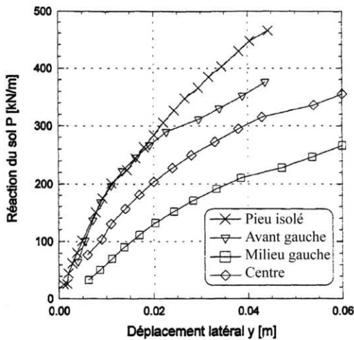
Figure 3. Courbes P-y obtenues par des essais en centrifugeuse sur un pieu isolé et les pieux au sein du groupe associé de 3x3 pieux de 3 diamètres d'entre-axe selon leur position (Remaud, 1999).
