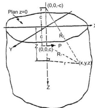
Figure 5. Force parallèle à la frontière à l'intérieur d'un massif semi-infini. (X, Y, Z) représente le repère dans lequel sont exprimées les équations (Mindlin, 1936)
