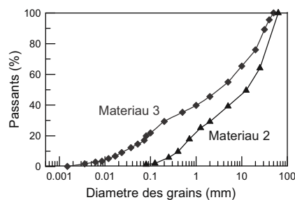
Figure 1. Courbes granulométriques des matériaux étudiés
