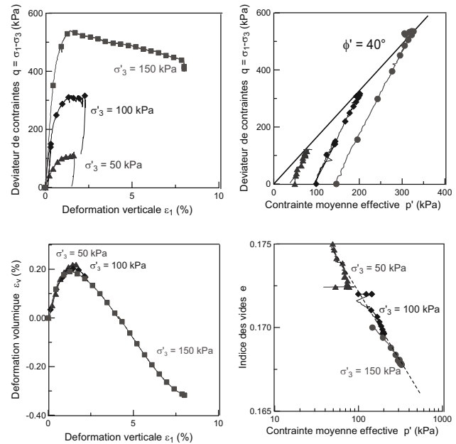
Figure 3. Résultats des essais triaxiaux multi-stage sur le matériau n° 2
