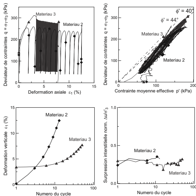
Figure 4. Résultats des essais cycliques sur les matériaux 2 et 3 ( \sigma'_{3c} = 70 kPa, \sigma'_{1c} = 200 kPa q_c/\sigma'_{3c} = \pm 1.6 )
