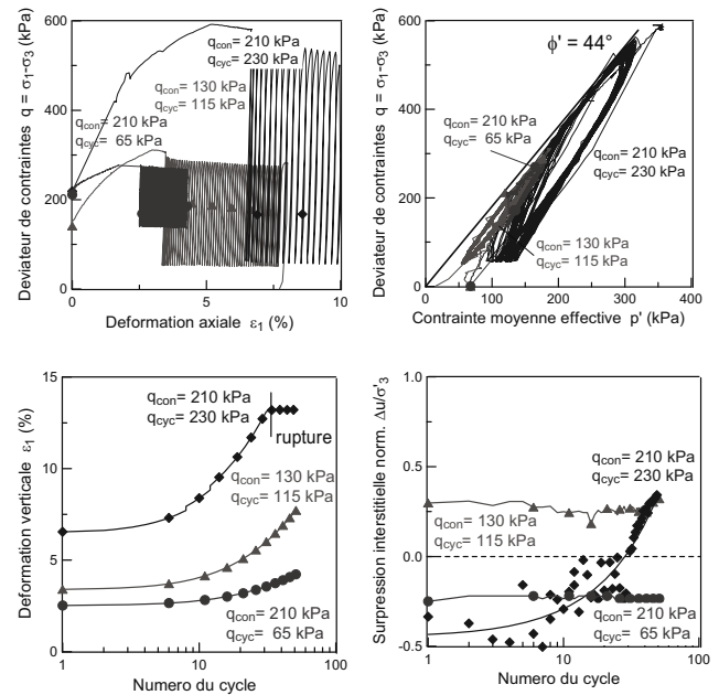
Figure 5. Essais sous différents déviateurs cycliques (matériau 3, \sigma'_{3c} = 70 kPa, q_c/\sigma'_{3c} = 1, 1.6 et 3.4 )
