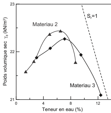
Figure 2. Courbes de compactage des matériaux étudiés
