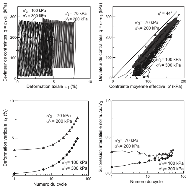
Figure 6. Essais sur des échantillons préparés à différentes contraintes de consolidation (matériau 3, q_c = 125 et 115 kPa)
