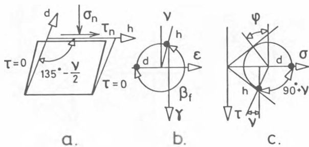
Fig. 9 Simple shear
