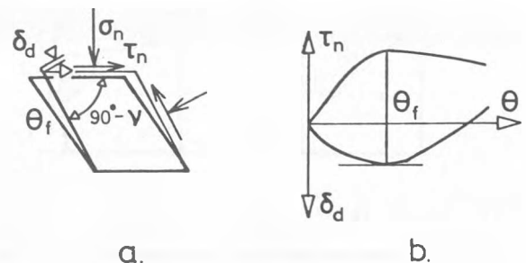
Fig. 8 Pure shear
