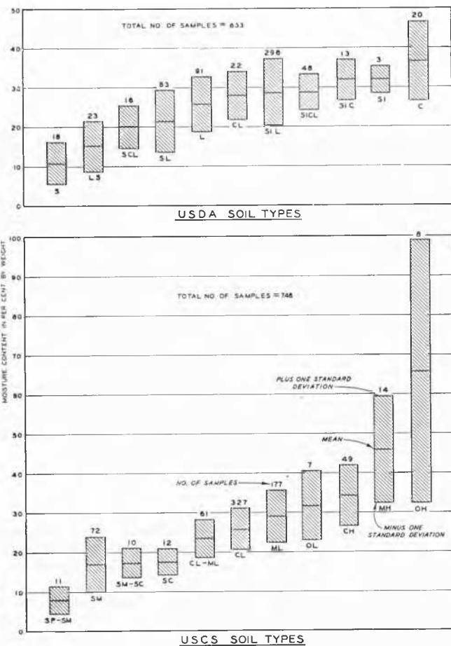
Fig. 1 Field maximum moisture contents, means and ranges. Teneurs en eau maxima du terrain, moyennes et valeurs limites.
