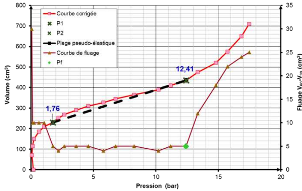
Figure 6. Exemple d'un résultat d'essai pressiométrique Ménard classique.
