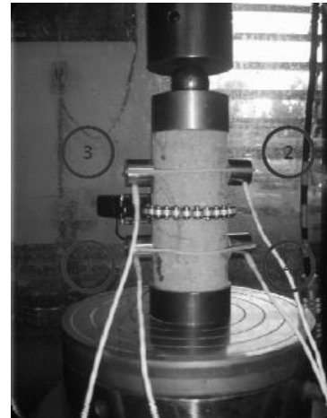
Figura 6. Cuerpo de prueba cilíndrico extraído de cuerpo de prueba prismático monitoreado con 4 sensores de emisión acústica y un extensómetro radial.
