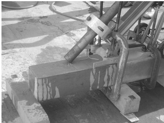
Figura 5. Esquema del equipo para la extracción de los cuerpos cilíndricos con inclinación de 45° en cuerpos prismáticos.
