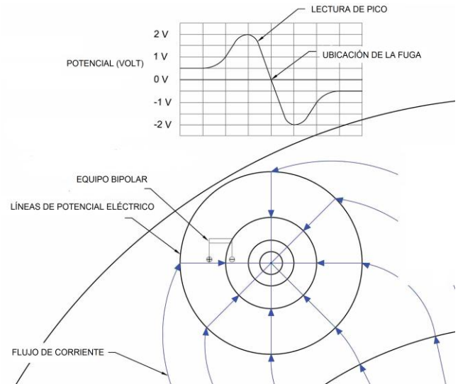
Figura 3. Ocurrencia de fuga en el método bipolar
