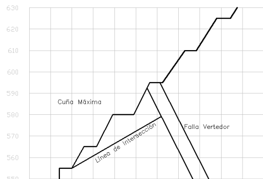
Figura 8. Sección a través de la línea de intersección de la cuña.
