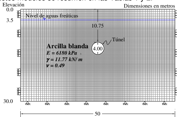
Figura 6. Modelo bidimensional de diferencias finitas
