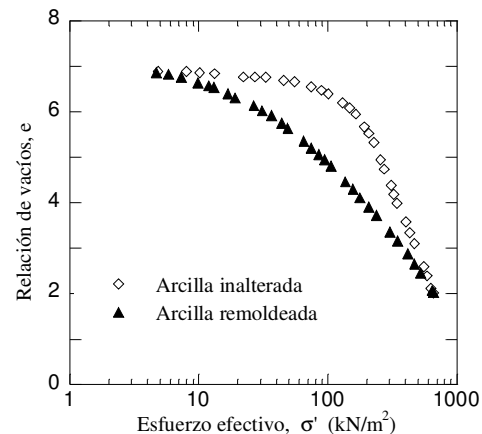
Figura 5. Efecto del remoldeo en la compresibilidad de arcillas de la ciudad de México (modificado de Romo, 1985)
