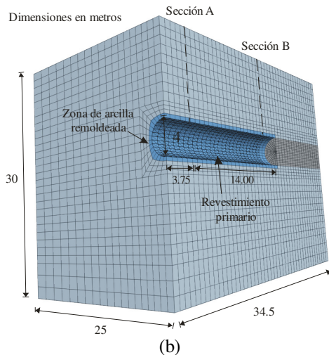
Figura 11. Modelo tridimensional de diferencias finitas La Figura 11 muestra la zona remoldeada alrededor del túnel. Este efecto se simuló cambiando las propiedades de la arcilla obtenidas del modelo Cam clay modificado de muestras inalteradas, como se explicó en la sección 4.1.4, por las obtenidas considerando las curvas de compresibilidad correspondientes a la arcilla remoldeada, que se presentan en la Figura 10.
