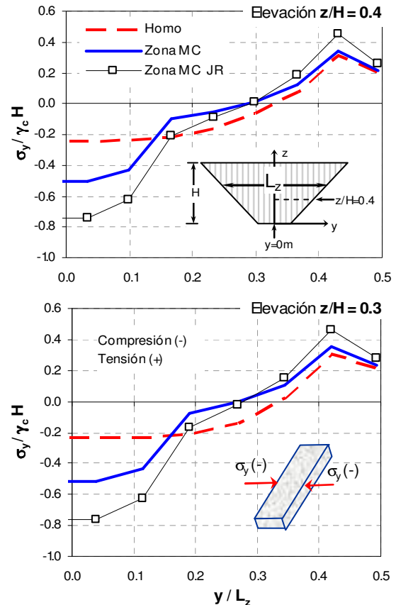
Figura 7. Esfuerzos transversales a lo largo de dos ejes horizontales al final del llenado del embalse.
