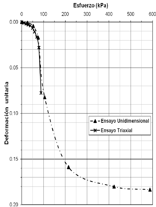
Figura 2. Gráficas esfuerzo-deformación unitaria obtenida en los ensayos de colapso
