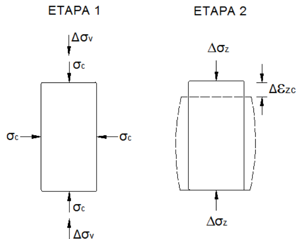
Figura 1. Ensayo de colapso en cámara triaxial
