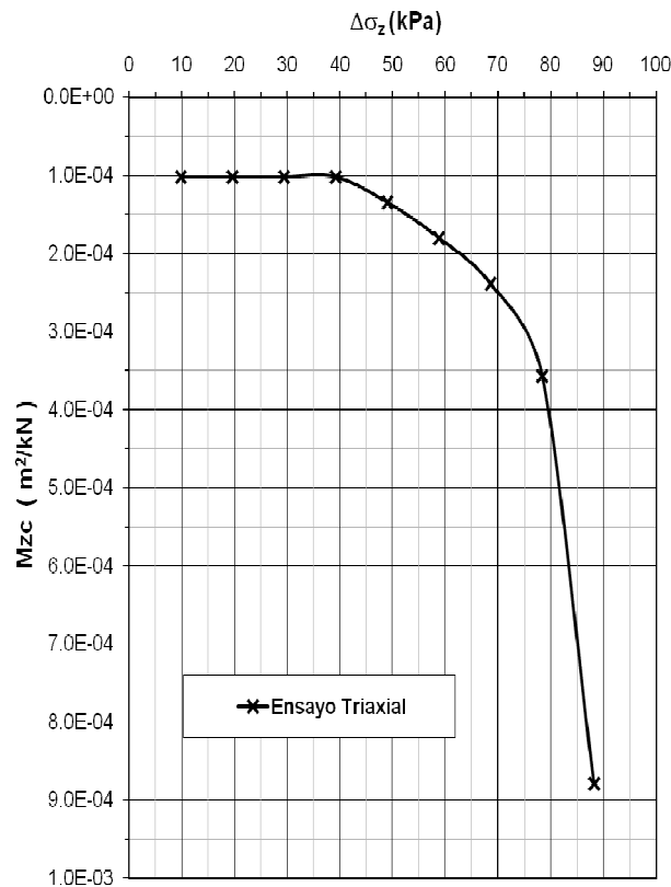
Figura 5. Gráfica \Delta\sigma_z - M_{zc} correspondiente al ensayo triaxial
