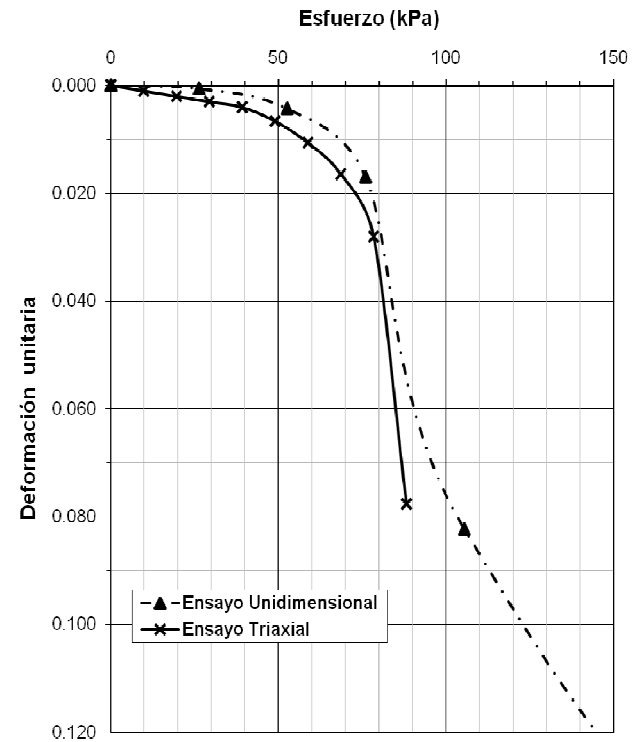
Figura 3. Detalle de la gráfica esfuerzo deformación unitaria (Figura 2) obtenida en los ensayos de colapso
