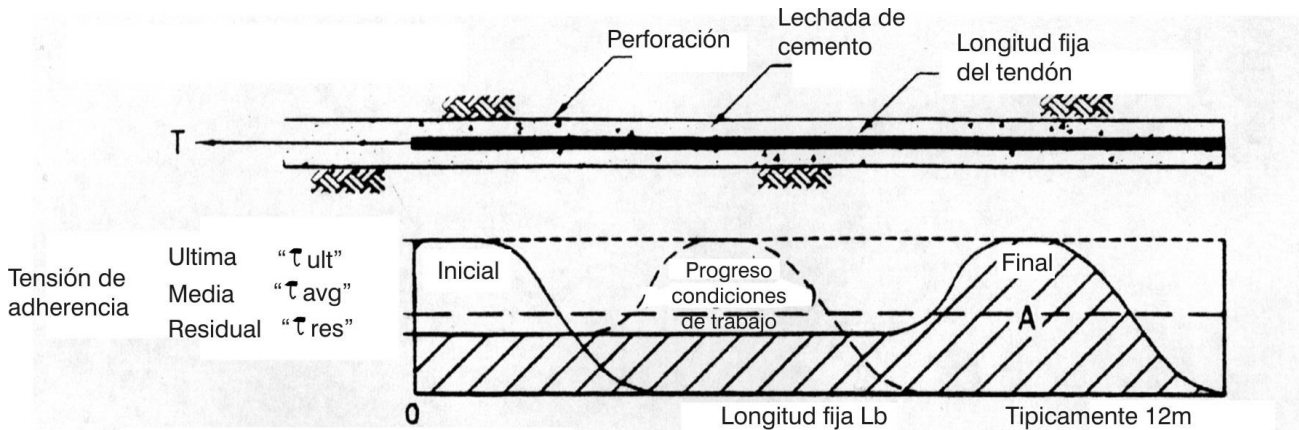
Figura 8. Distribución de tensiones de adherencia en la longitud fija, para distintas etapas de un ensayo de carga hasta llegar a la rotura. El área A constituye la carga máxima de la longitud fija del anclaje (Barley y Ostermayer, 2003).
