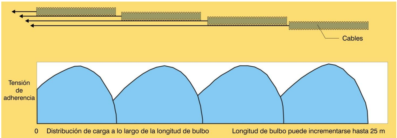
Figura 7. Distribución de tensiones de adherencias para varias unidades de anclajes eficientes (Fernández Vincent, 2005).
