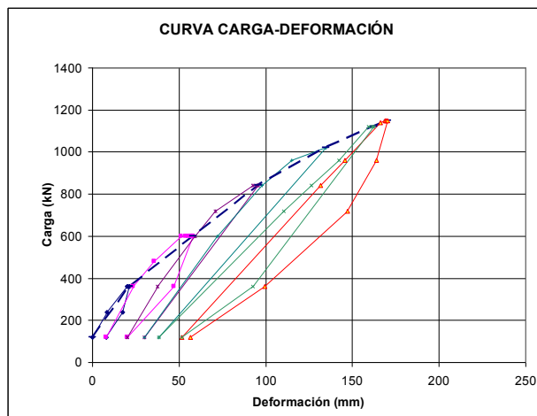
Figura 5. Ensayo de investigación anclaje TA1.
