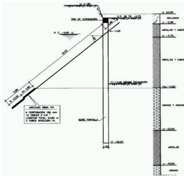
Figura 4. Ensayo de investigación anclaje TA1.
