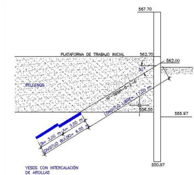
Figura 2. Sección tipo ensayos de investigación.
