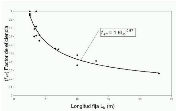
Figura 1. El factor de eficiencia vs. longitud fija (Barley, 1997).
