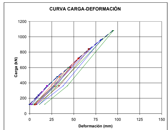
Figura 3. Ensayo unidad TA2-A.
