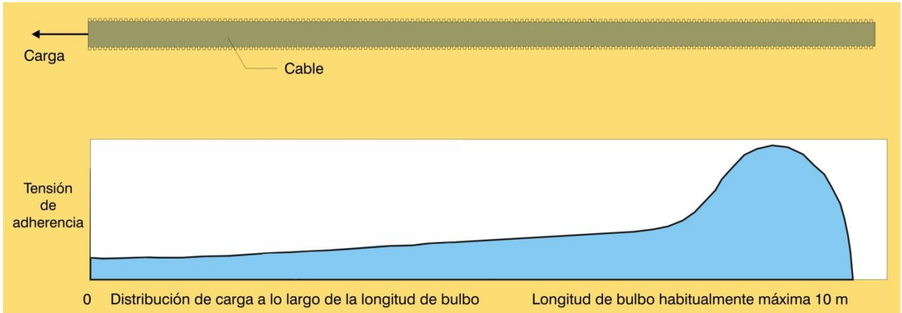
Figura 6. Distribución de tensiones de adherencia para la carga de rotura en un anclaje tradicional (Fernández Vincent, 2005).
