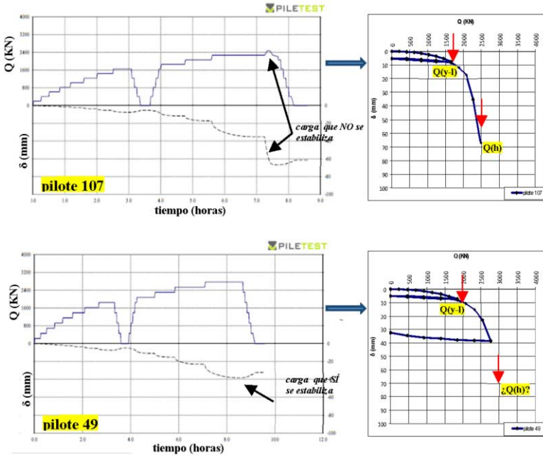
Figura 2. Ensayo de carga estática en dos pilotes.
