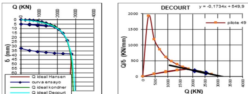
Figura 3. Interpretación del ensayo del pilote 49 con los tres Métodos de extrapolación descritos.
