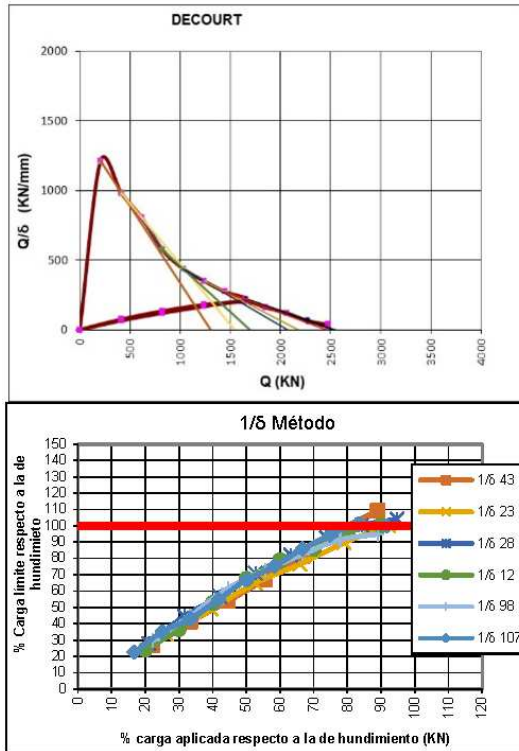
Figura 7. Posibles extrapolaciones en fase al recorrido del ensayo.
