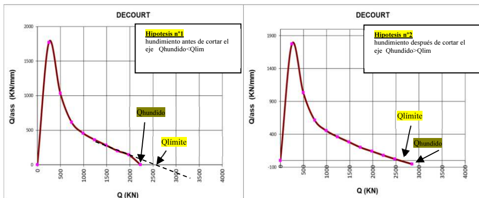
Figura 5. Posibles cargas interpretadas de hundimiento en un ensayo real.
