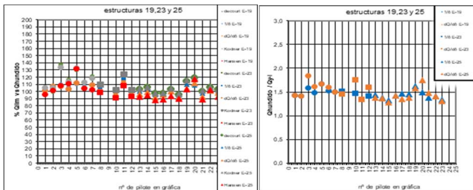
Figura 6. Relaciones entre la Qlim y Qh; así como la Qh y la Qy-1.
