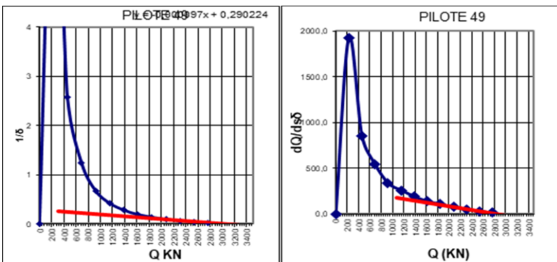
Figura 4. Ensayo del pilote 49. Métodos de extrapolación y determinación de inicio de la fluencia.
