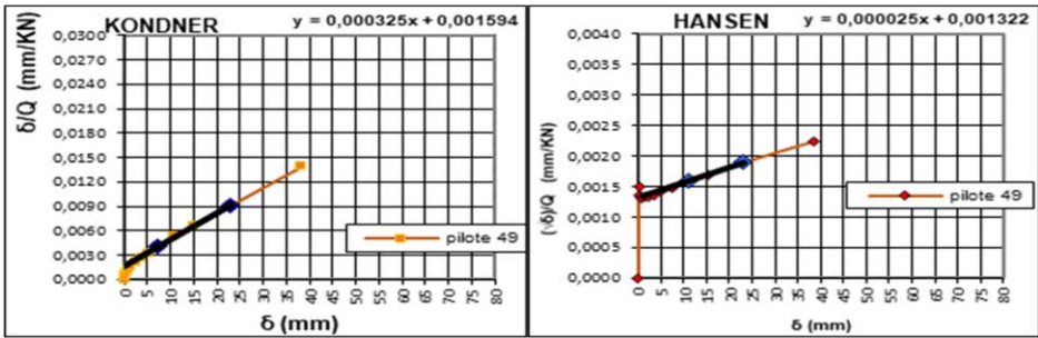
Figura 3. (continuación) Interpretación del ensayo del pilote 49 con los tres Métodos de extrapolación descritos.
