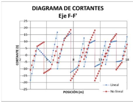
Figura 8. Diagramas de cortante, eje F-F'.
