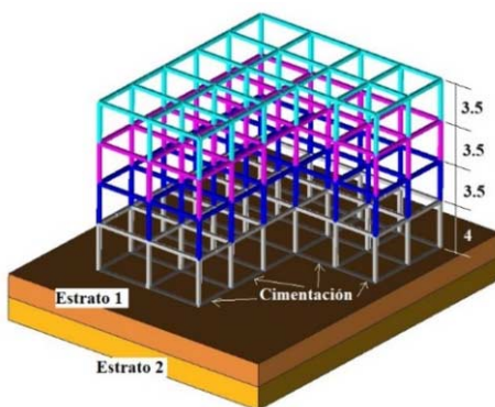
Figura 3. Modelo del edificio y cimentación sobre dos estratos de suelo friccionante. Cotitas en metros.
