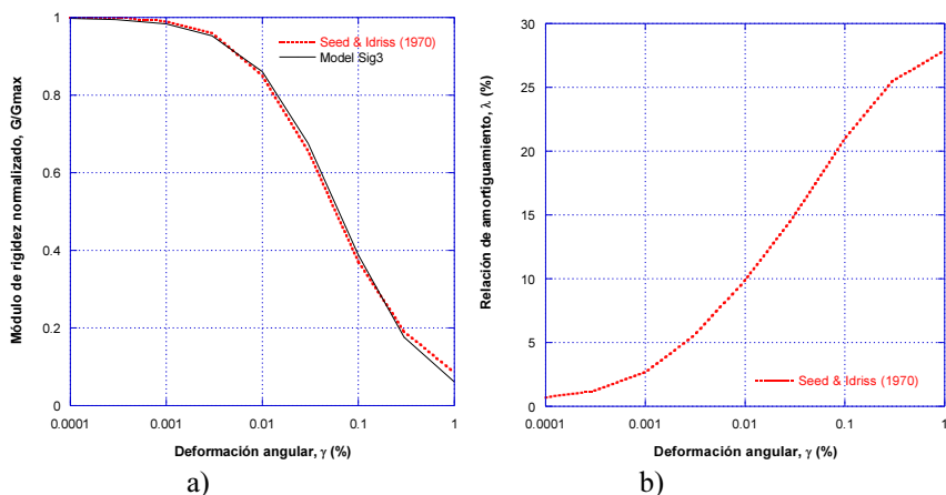
Figura 5. (a) Curva del módulo de rigidez normalizado y (b) curva de amortiguamiento, utilizadas en el análisis.
