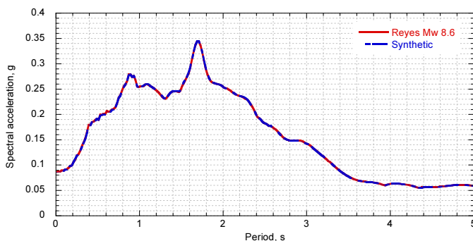
Figura 7. Espectros de respuesta (Reyes 1999) y espectro de respuesta ajustado para una magnitud M_w de 8.6.
