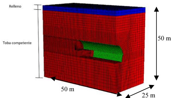
Figura 6. Modelo numérico desarrollado.
