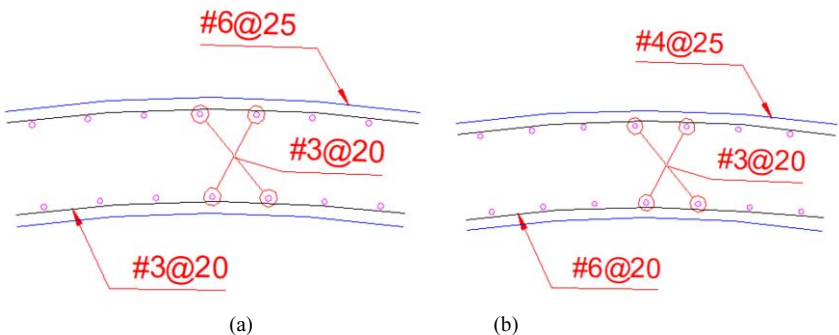
Figura 3. Detalle de construcción del revestimiento secundario del túnel (a) Hastiales y (b) Bóveda.
