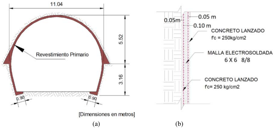
Figura 2. (a) Sección transversal del túnel y (b) Sección del revestimiento primario.
