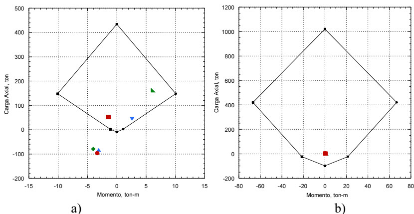
Figura 8. Diagrama de interacción (a) revestimiento primario and (b) revestimiento secundario.
