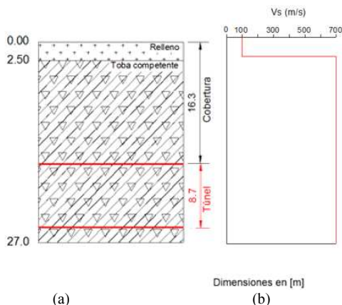
Figura 4. a) Perfil del suelo de la sección analizada, y b) Perfil de la velocidad de onda de corte.
