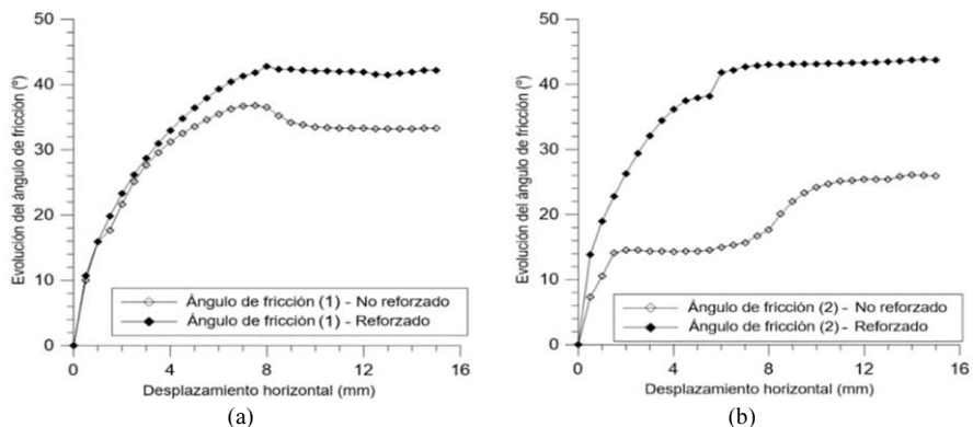
Figura 6. Evolución del ángulo de fricción: (a) Esfuerzos bajos - 25, 50 y 100 kPa, (b) Esfuerzos altos - 200 y 400 kPa.
