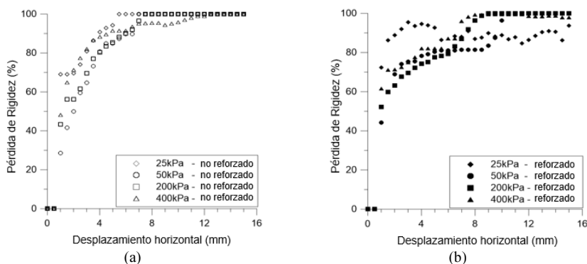
Figura 4. Evolución de la pérdida de rigidez inicial: (a) Relave no reforzado (b) Relave reforzado.
