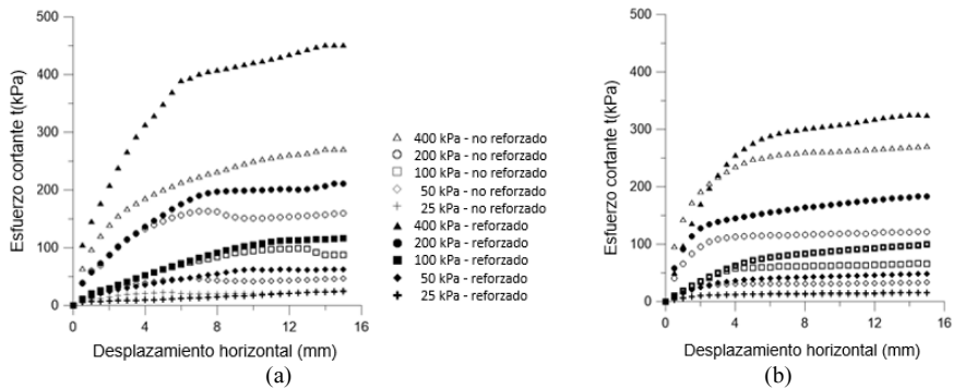
Figura 3. Curvas esfuerzo cortante - desplazamiento horizontal. (a) ensayo convencional (b) ensayo de plano cortado con superficie pulida.
