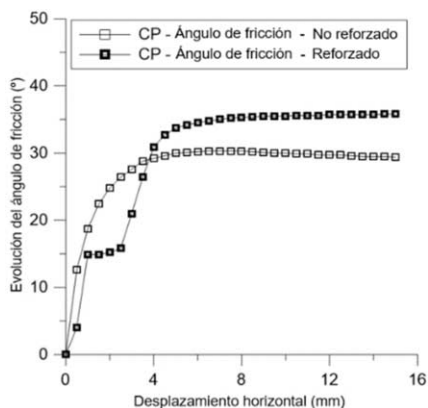
Figura 8. Evolución del ángulo de fricción. Ensayo de plano cortado con superficie pulida.
