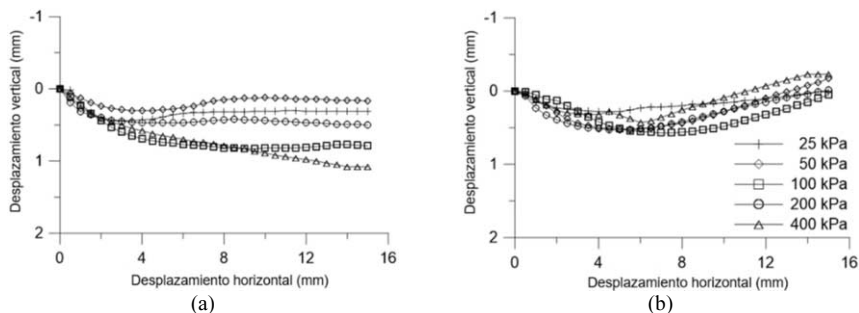
Figura 9. Variación volumétrica: Ensayo convencional: (a) no reforzada (b) reforzada.
