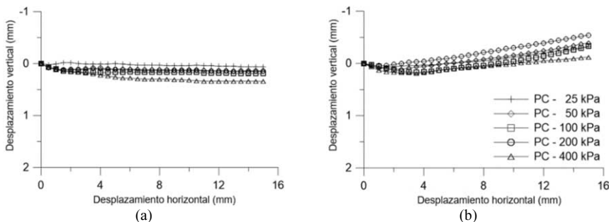
Figura 10. Variación volumétrica: Ensayo de plano cortado con superficie pulida: (a) no reforzada, (b) reforzada.
