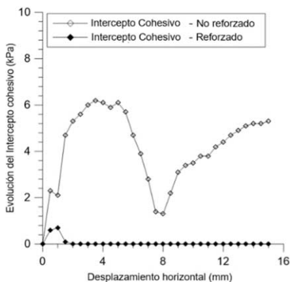
Figura 7. Evolución del intercepto cohesivo. Ensayo convencional.
