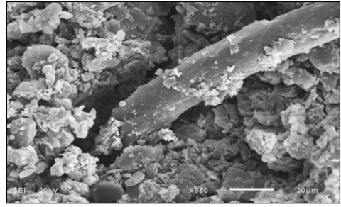
Figura 2. Interacción fibra-relave.
