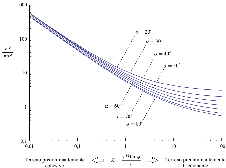
Figura B-1. Diagrama adimensional de estabilidad para la estimación del factor de seguridad normalizado obtenido con las ecuaciones (B-1) a (B-3).
