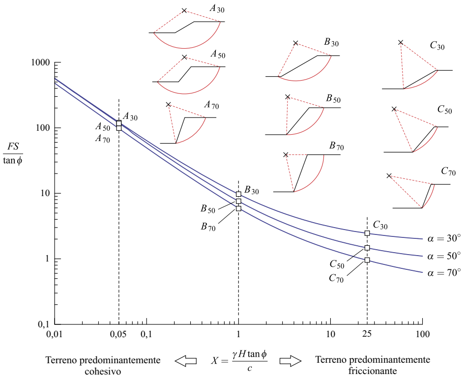
Figura 3. Diagrama adimensional de estabilidad que muestra la similitud de factor de seguridad normalizado y la posición de la superficie de falla crítica.
