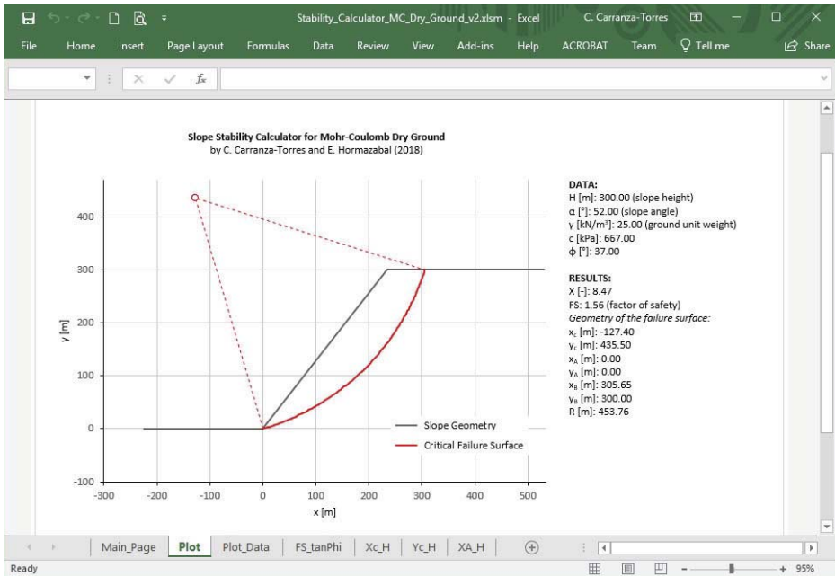
Figura 6. Hoja de cálculo gráfica en EXCEL que muestra la representación del problema de talud analizado.
