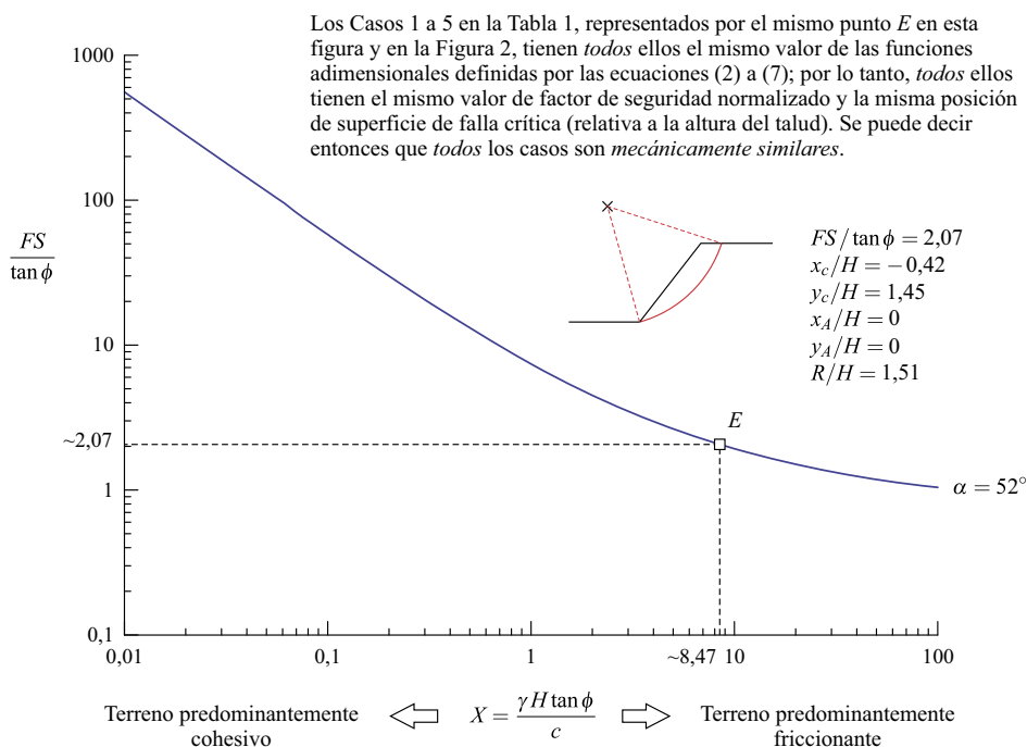
Figura 4. Diagrama adimensional de estabilidad que muestra la similitud de factor de seguridad y la posición de la superficie de falla crítica, para los casos listados en la Tabla 1.
