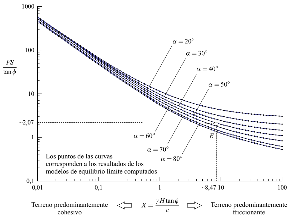
Figura 2. Diagrama adimensional para la estimación del factor de seguridad normalizado.
