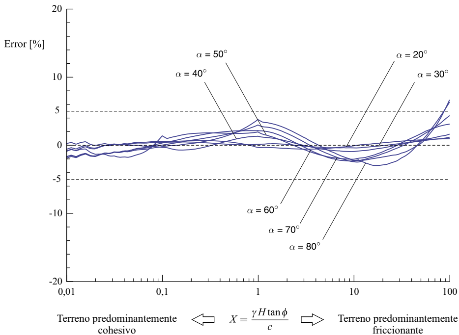
Figura B-2. Representación gráfica del error del factor de seguridad normalizado, calculado con la ecuación (B-4).
