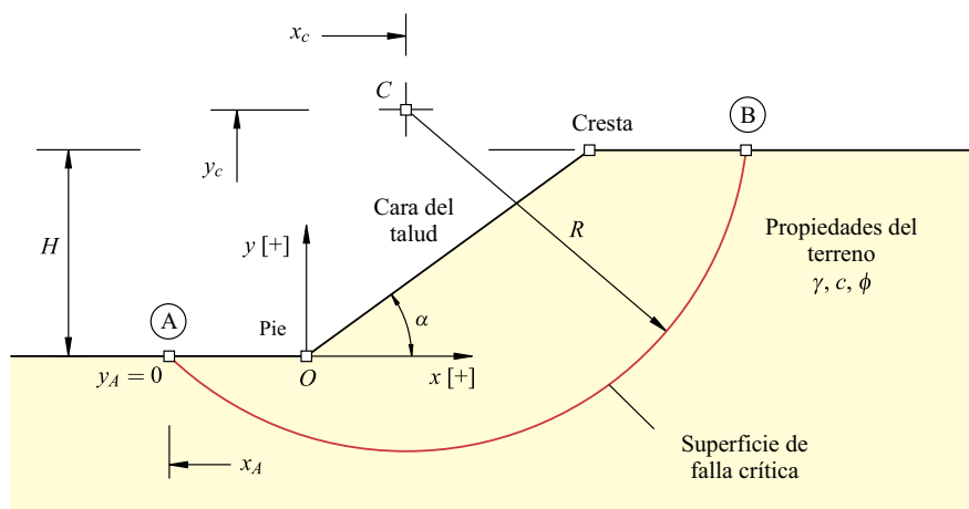
Figura 1. Talud en terreno seco que obedece el criterio de resistencia al corte Mohr-Coulomb.
