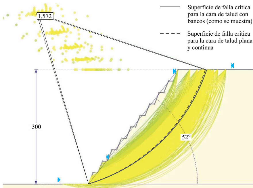
Figura 8. Modelo de equilibrio límite SLIDE (Rocscience Inc. [25]) para una sección de la mina a cielo abierto mostrada en la Figura 7.
